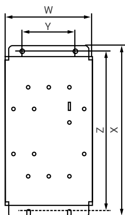
BASEPLATE A
